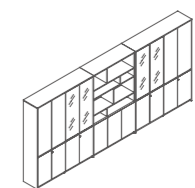
E99-2 W4364*D400*H2005(mm)
