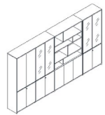
E98L-2 W3579*D400*H2005(mm)
